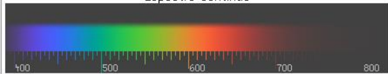
Espectro Contínuo
